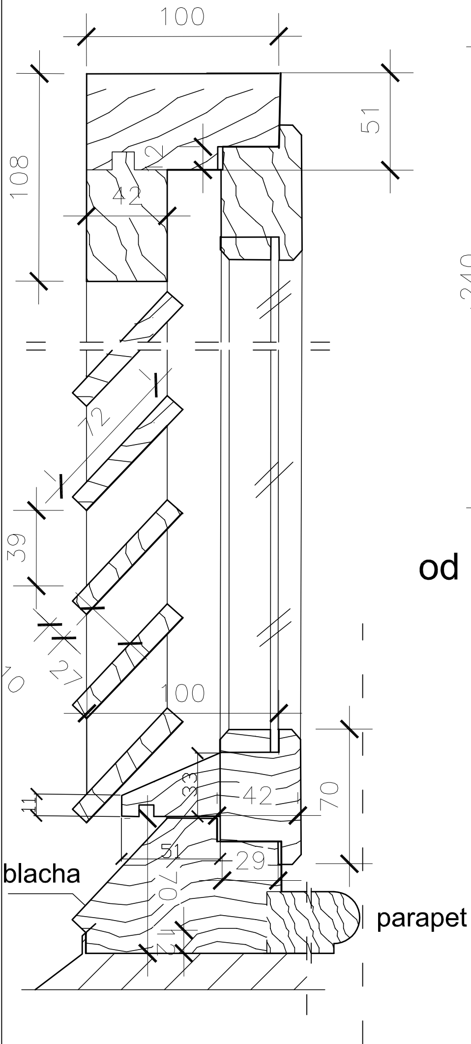
Detal A- przekrój pionowy
